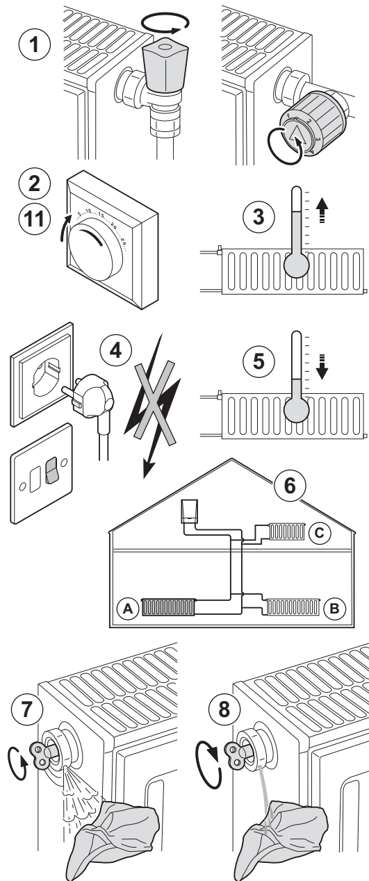
Afb.52 Ontluchten van de installatie
