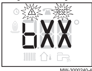
Afb.53 Weergave van storingscode
